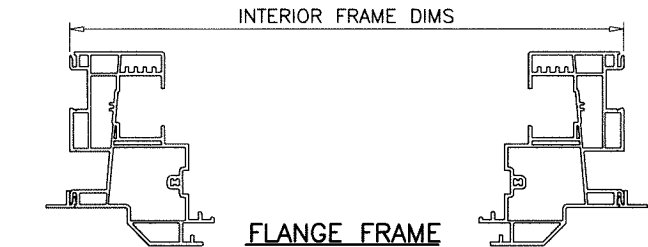
FLANGE FRAME
